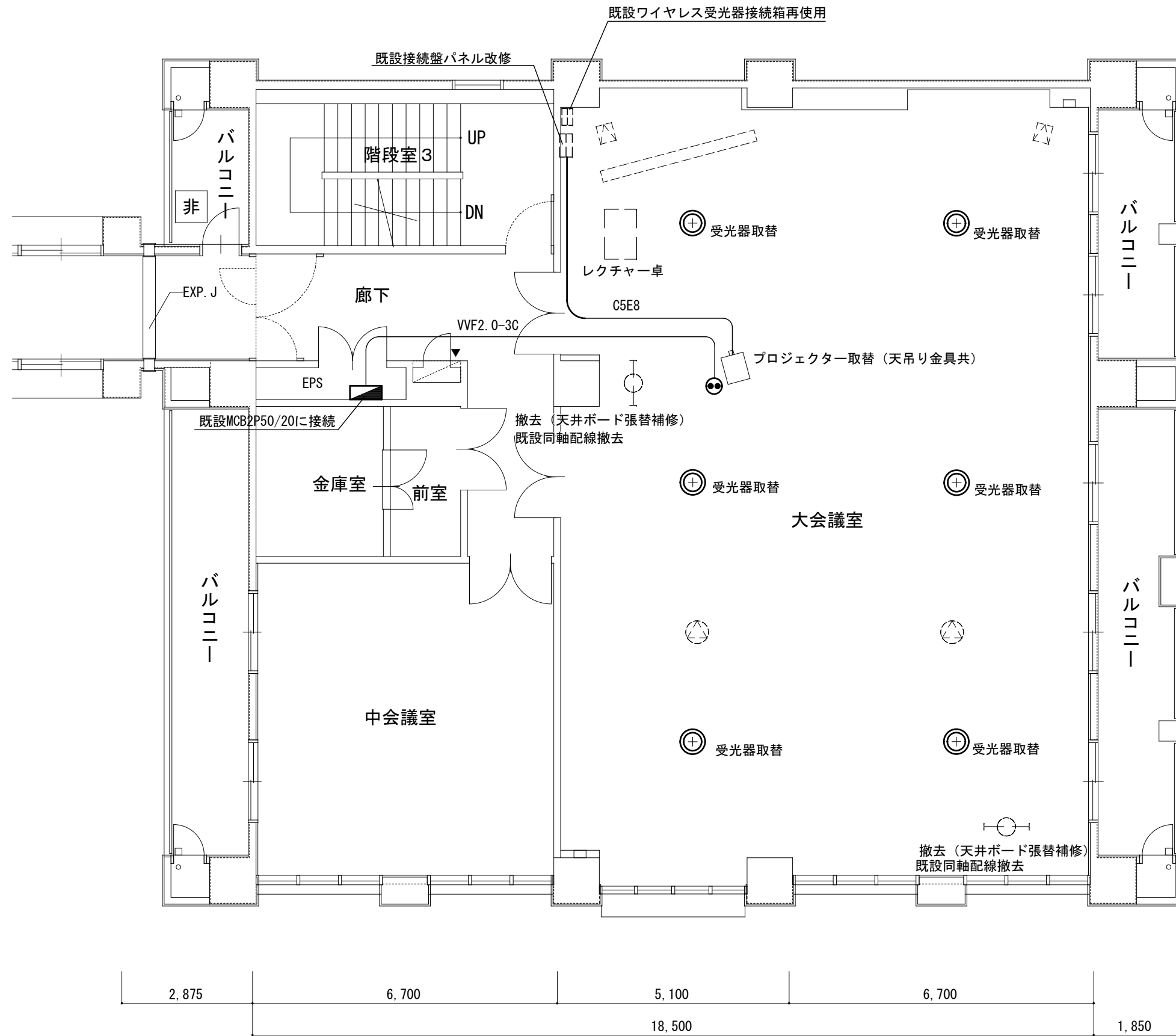
管理棟Ⅱ5階平面図
